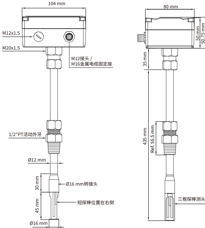
FTM94 (风管型)
