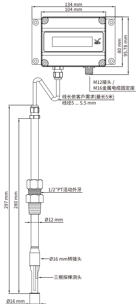
FTM95 (分离型)
